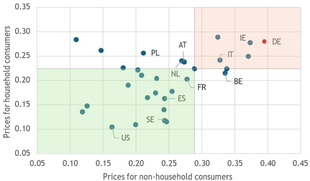
Gráfico 2: Precios de la electricidad doméstica y no doméstica, EUR/kWh
